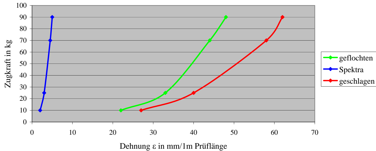
Dehnung der Leine in mm bezogen auf die Prüflänge von 1 m abhängig von der Zugkraft in kg
